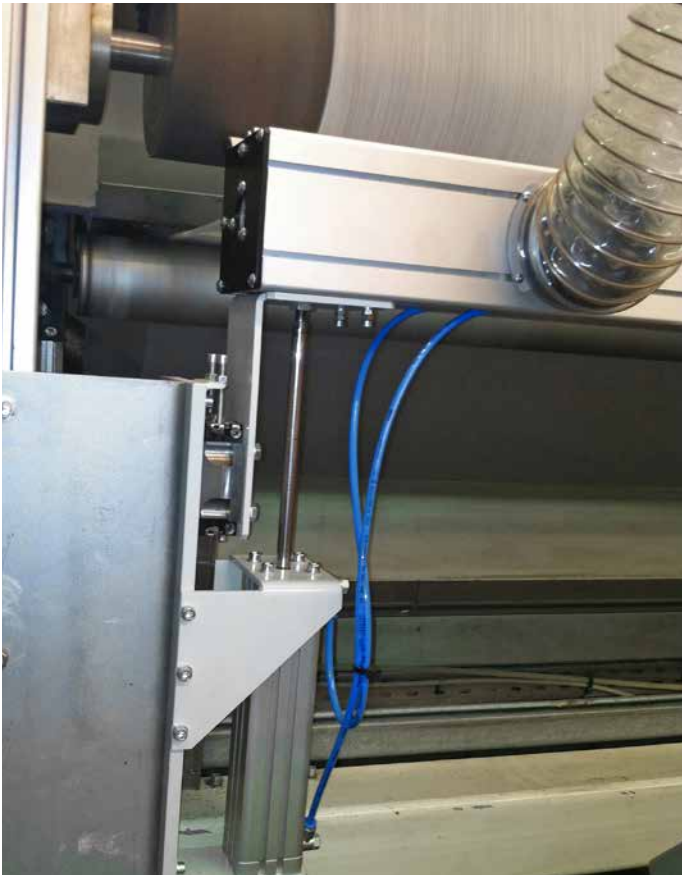
Absaugkopf mit Linearführung Suctionhead with linear guide
