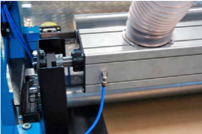
Absaugkopf mit Linearführung Suctionhead with linear guide
