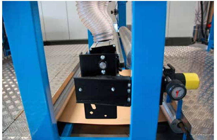
Distanzeinstellung und Positionsanzeige Distance setting and position display
