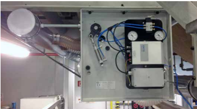
Trägerplatte mit Ionisationsgenerator Mounting plate with ionisation-generator
